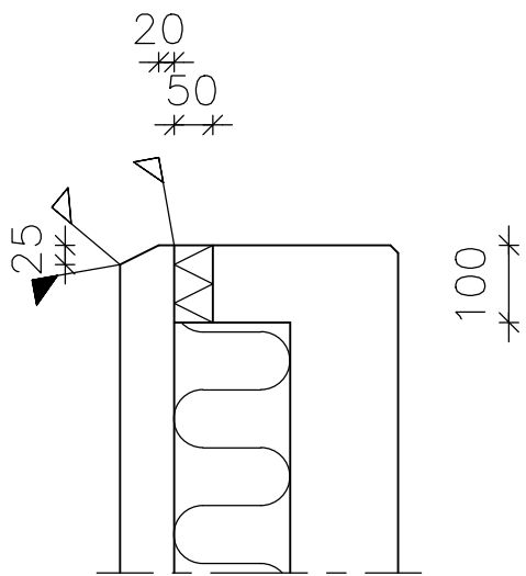
LODRET SNIT
